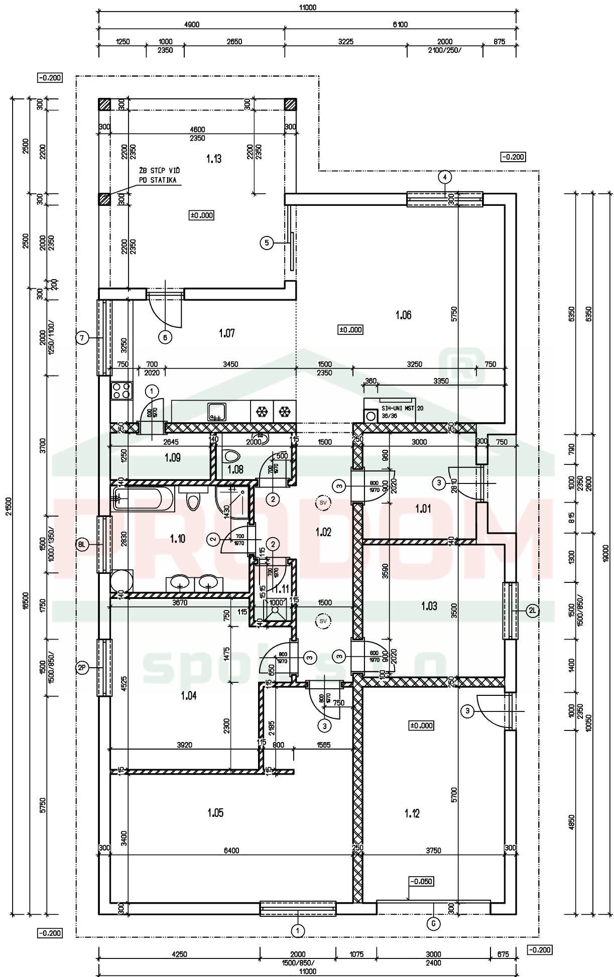
BUNGALOW 180
